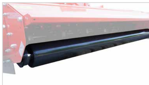
El rodillo de 135mm de diámetro incorpora rascador integrado y realiza el seguimiento del terreno.
