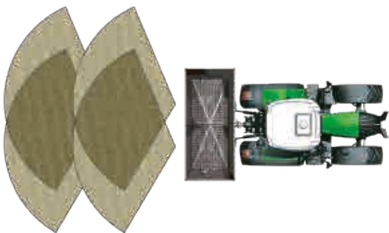
Concurrents: 2 pales par disque (Une mauvaise répartition des engrais en pente est causée par un changement du point de chute de l'engrais sur les disques)
